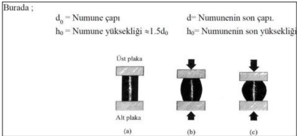
Şekil 2. Basma Kuvveti uygulanan sünek malzemelerdeki fiçı oluşumu; a) basma kuvveti yok, b) Basma kuvveti etkisiyle fiçı oluşumunun ilk aşaması, c) Fıçı oluşumunun tamamlanması
