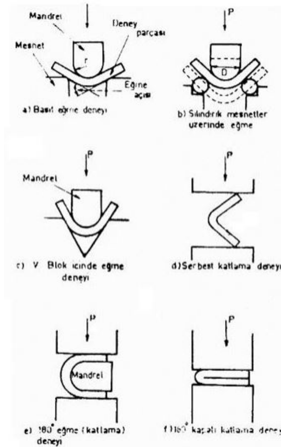
Şekil 8. Değişik eğme deneyi düzenekleri
