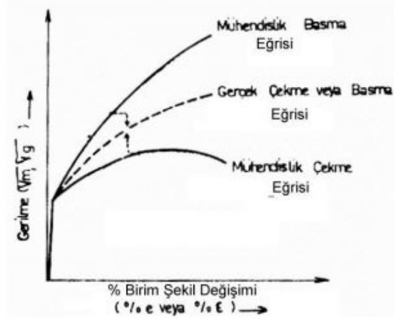
Şekil 4. Metalik bir malzemenin mühendislik (teknolojik) ve gerçək çekme-basma diyagramlarının şematik gösterimi
