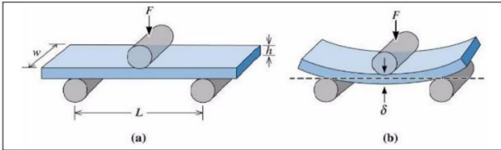
Şekil 7. Üç nokta eğme deneyinin şematik gösterimi
