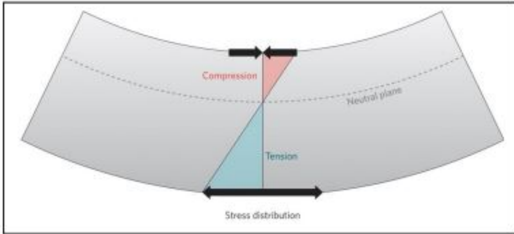
Şekil 6. Eğilme halindeki çubuk üzerindeki gerilme dağılımı
